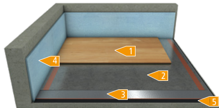
Fußbodenheizung (schwimmend)
