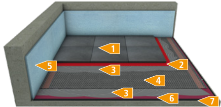
Fußbodenheizung (verklebt)
