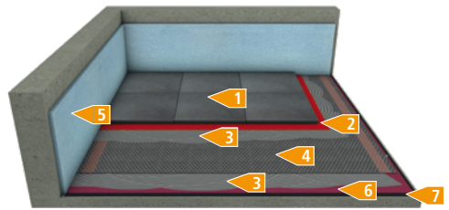
Fußbodenheizung (verklebt)
