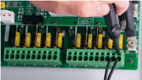
Ausgangsklemmen 24 V (2,5 mm 2 – 6,0 mm 2 )
