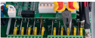
Heizkreissicherung austauschen
