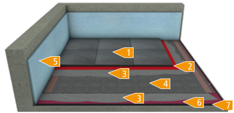
Fußbodenheizung (verklebt)
